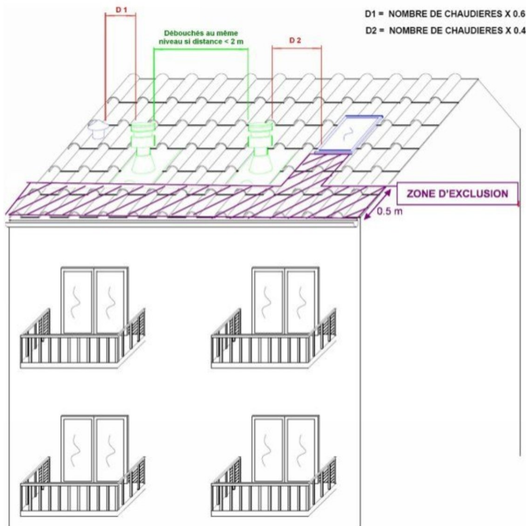
Figure 2 – Principe de positionnement des terminaux
