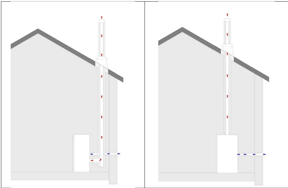
Figure 2c- configuration avec terminal vertical (conduit en situation intérieure)
