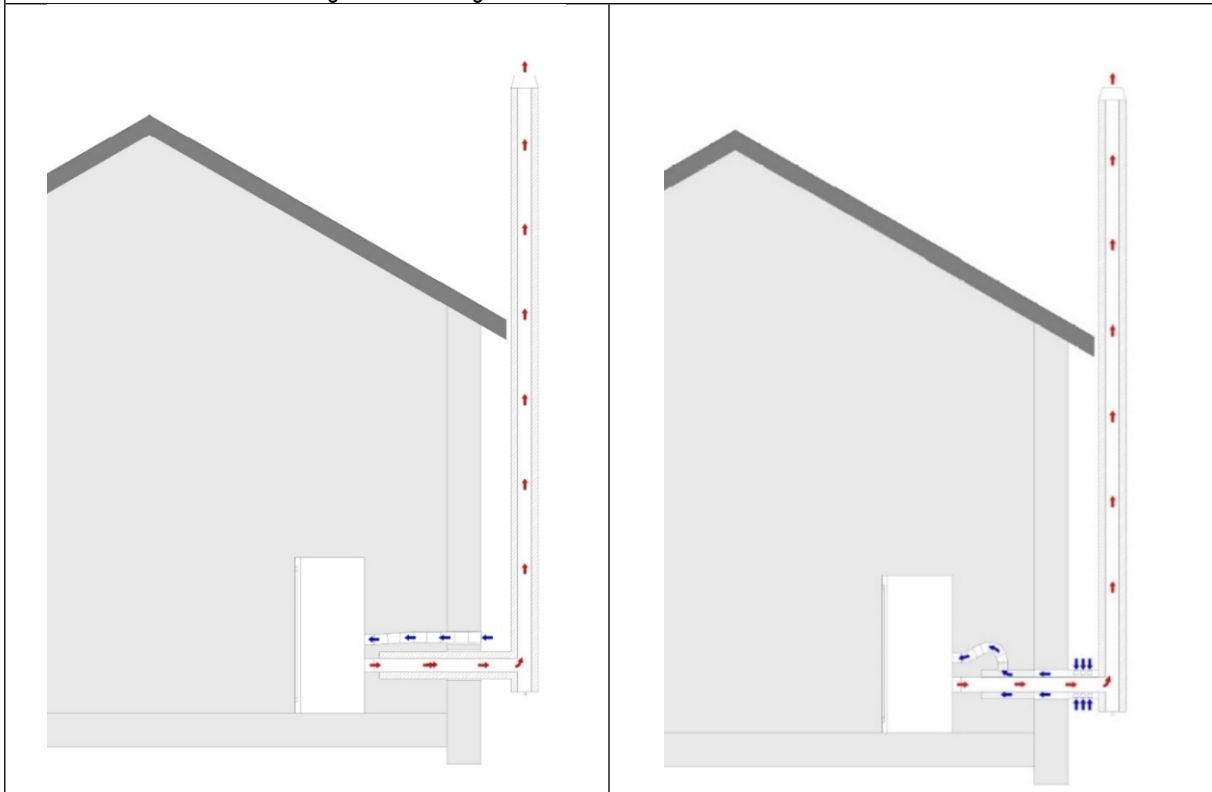
Figure 2b – configuration avec terminal vertical (conduit en situation extérieure)
