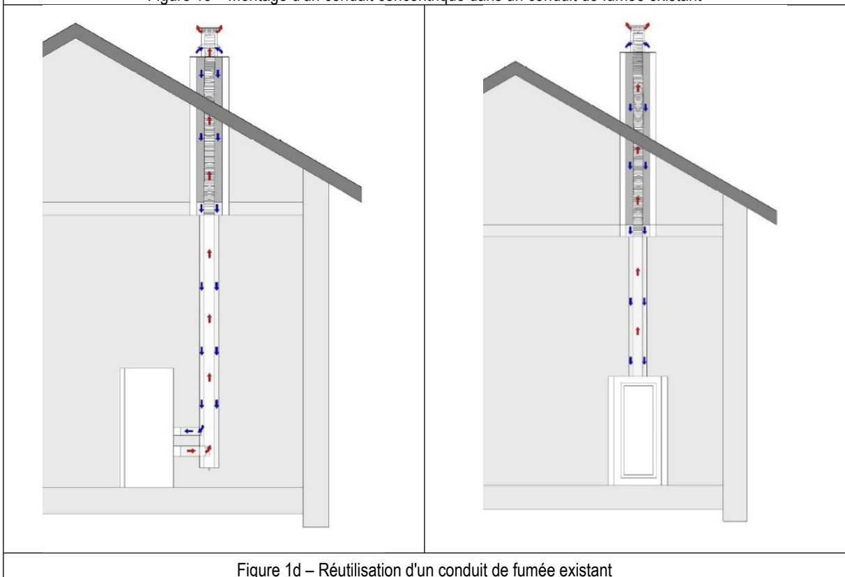
Figure 1 – Schémas de principe - configurations avec terminaux concentriques
