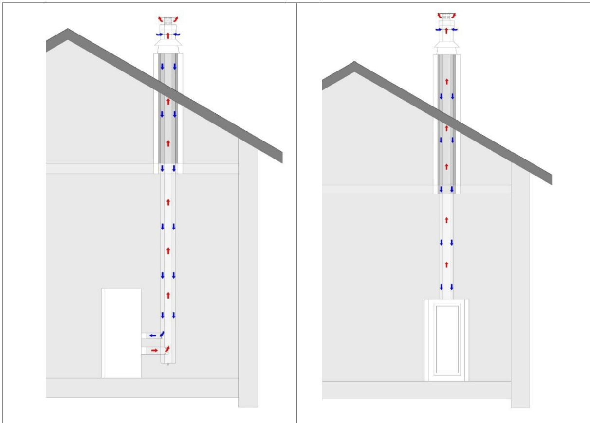
Figure 1c – Montage d'un conduit concentrique dans un conduit de fumée existant
